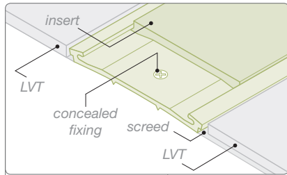
ELACS5040 LVT to LVT.
