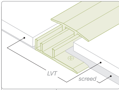
KC578 LVT to LVT.
